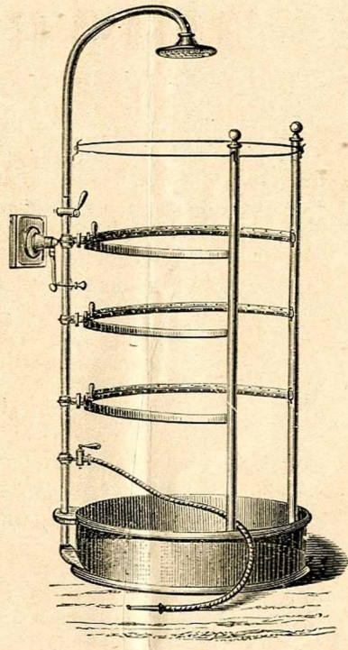
N° 13. Appareil d'hydrothérapie pour appartements et salles de bains s'adaptant à une prise d'eau avec pression. Il est composé d'une douche en pluie, douche locale avec lance à 2 jets à spatule, de deux pommes d'arrosoir et de trois cercles à trois rangées de trous, d'un bassin de 80 centimètres de diamètre. Hauteur de l'appareil, 2 m 40 ..... 300 »
