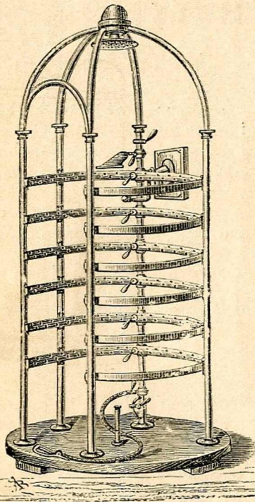
N° 12. Appareil pour salle de bains, grand modèle, s'adaptant à une prise d'eau avec pression. Il est composé de 6 cercles à trois rangées de trous, d'une douche en pluie, douche oblique, douche ascendante avec siège et d'une doue locale avec lance à deux jets et éventails et de deux pommes d'arrosoir. Hauteur 2 m 50, diamètre 1 mètre. L'appareil est en cuivre poli monté sur un fond en chêne..... 900 »
