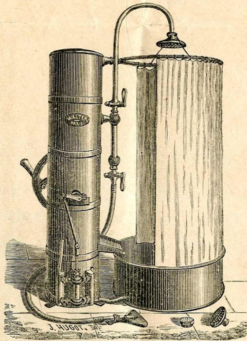
N° 7. Appareil pour Douches à pression d'air, de 2 m 40 de hauteur sur 1 m 30 de longueur et 82 cent. de largeur contenant 150 litres d'eau sous pression de 3 atmosphères, et composé de la douche en pluie, d'une douche locale mobile avec 2 pommes d'arrosoir, et lance à 2 jets à spatule, de la pompe à double effet et d'un manomètre. Son prix est de..... 350 »
