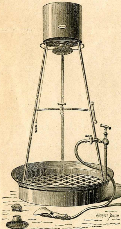
N° 5. Appareil pour Douches à pression d'air ayant 2 m 55 de hauteur sur 92 cent. de diamètre contenant 40 litres d'eau sous pression de 3 atmosphères, composé de la douche en pluie et d'une douche en jet mobile avec 2 pommes d'arrosoir et lance à 2 jets à spatules et d'une pomme à manomètre.. 220 »
