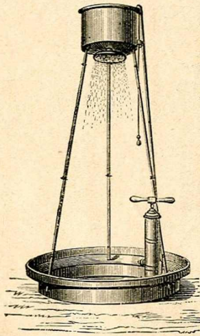
N° 10 Appareil pour Douches en pluie contenant 40 litres, avec pression du poids de l'eau, ayant 2 m 45 de hauteur sur 92 centimètres de diamètre ..... 100 »
